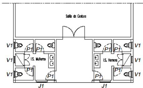
Planta do Piso
