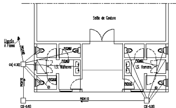
Planta do Piso - Rede de Esgotos
