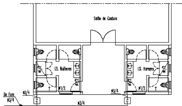
Planta do Piso - Rede Aguas
